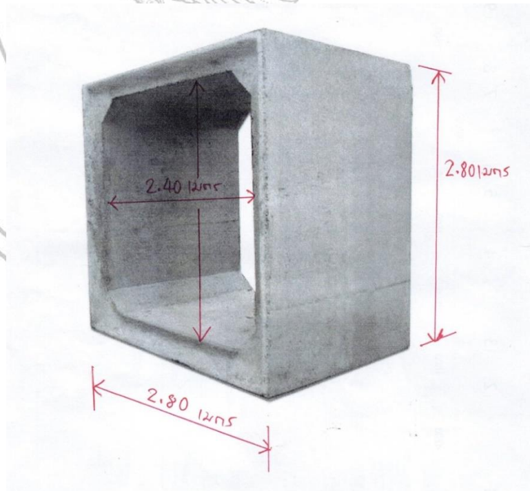
รูปภาพที่ 3 ท่อระบายน้ำคอนกรีตเสริมเหล็กขนาด 2.40 x 2.40 เมตร
